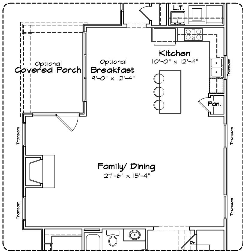
2 Optional Breakfast Scale: \frac{1}{8}'' = 1'-0'' Adds 58 s.f.
